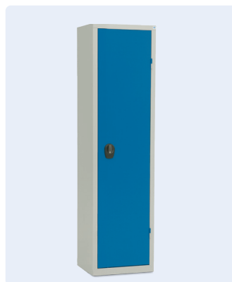
Artikelnr. 131V0095 MS-1 med enkel dörr och 4 galv. hyllor Utvändigt mått mm: H:2000 B:475 D:445 Karmmått i mm: H:1870 B:395 D:425
