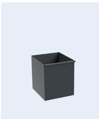
Artikelnr. 132B0025-B-7016 Behållare till avfallsskåp (142H0016-B-7016-7016) Utvändigt mått mm.: H:560 B:475 D:560/530
